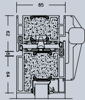
Snit C-C
