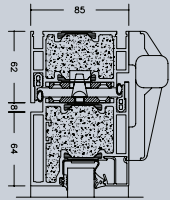
Snit A-A
