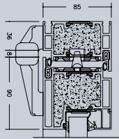
Snit G-G
