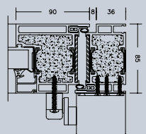
Snit F1-F1
