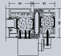
Snit D-D
