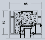
Snit C-C
