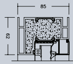
Snit A-A
